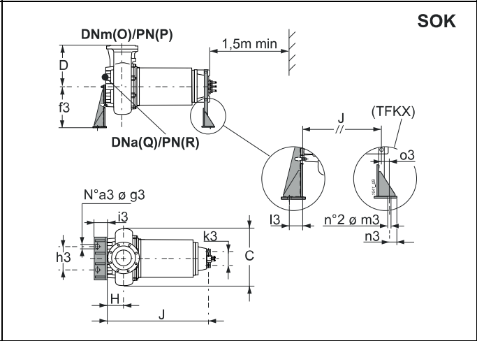
For fixed installation in a dry chamber - horizontal (/R) Versión para cámara seca - horizontal (/R) Esecuzione per camera asciutta - orizzontale (/R)
