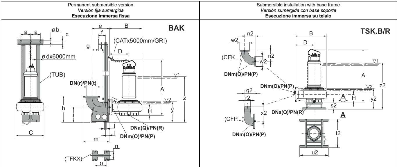
Permanent submersible version Versión fija sumergida Esecuzione immersa fissa
