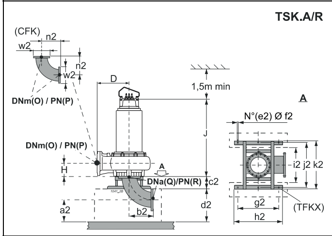
Permanent submersible version Versión fija sumergida Esecuzione immersa fissa
