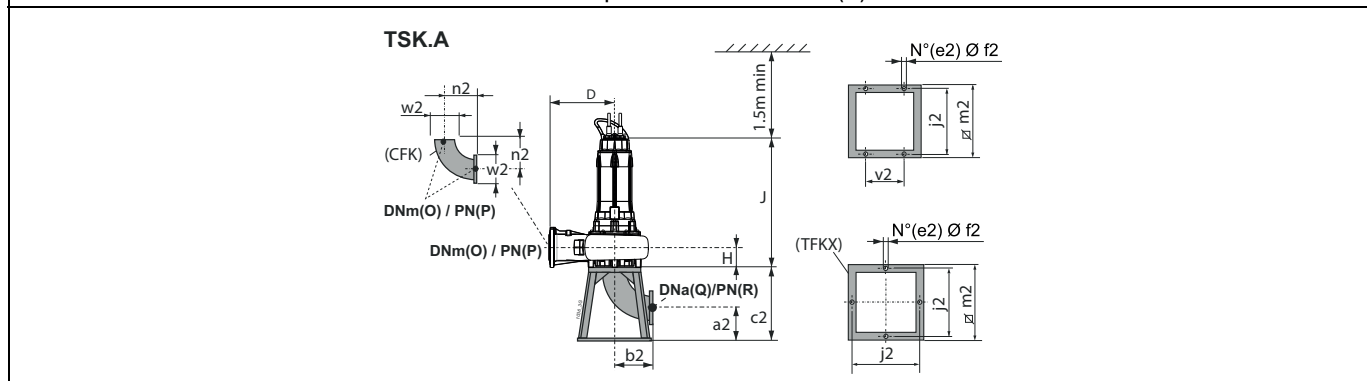
Version para cámara seca - vertical (/R) Für Trockeninstallation - senkrecht (/R) Esecuzione per camera asciutta - verticale (/R)
