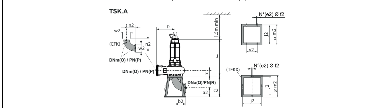
Versión para cámara seca - vertical (/R) Für Trockeninstallation - senkrecht (/R) Esecuzione per camera asciutta - verticale (/R)
