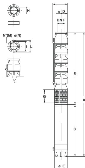
Overall dimensions and weights / Dimensions d'encombrement et poids Dimensioni di ingombro e pesi
