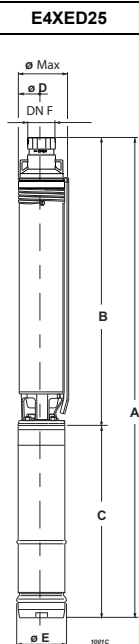
Overall dimensions and weights Dimensiones máximas y pesos Dimensioni di ingombro e pesi
