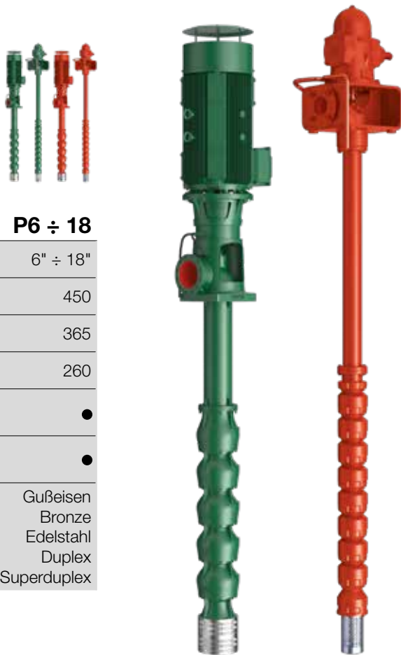
Antriebseinheit mit Elektromotor
