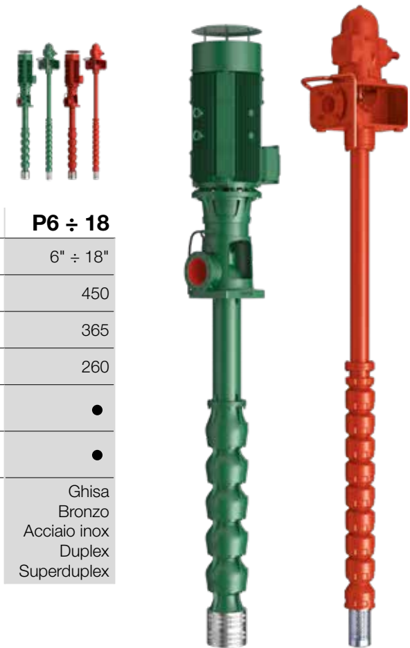
Gruppo di comando con motore elettrico
