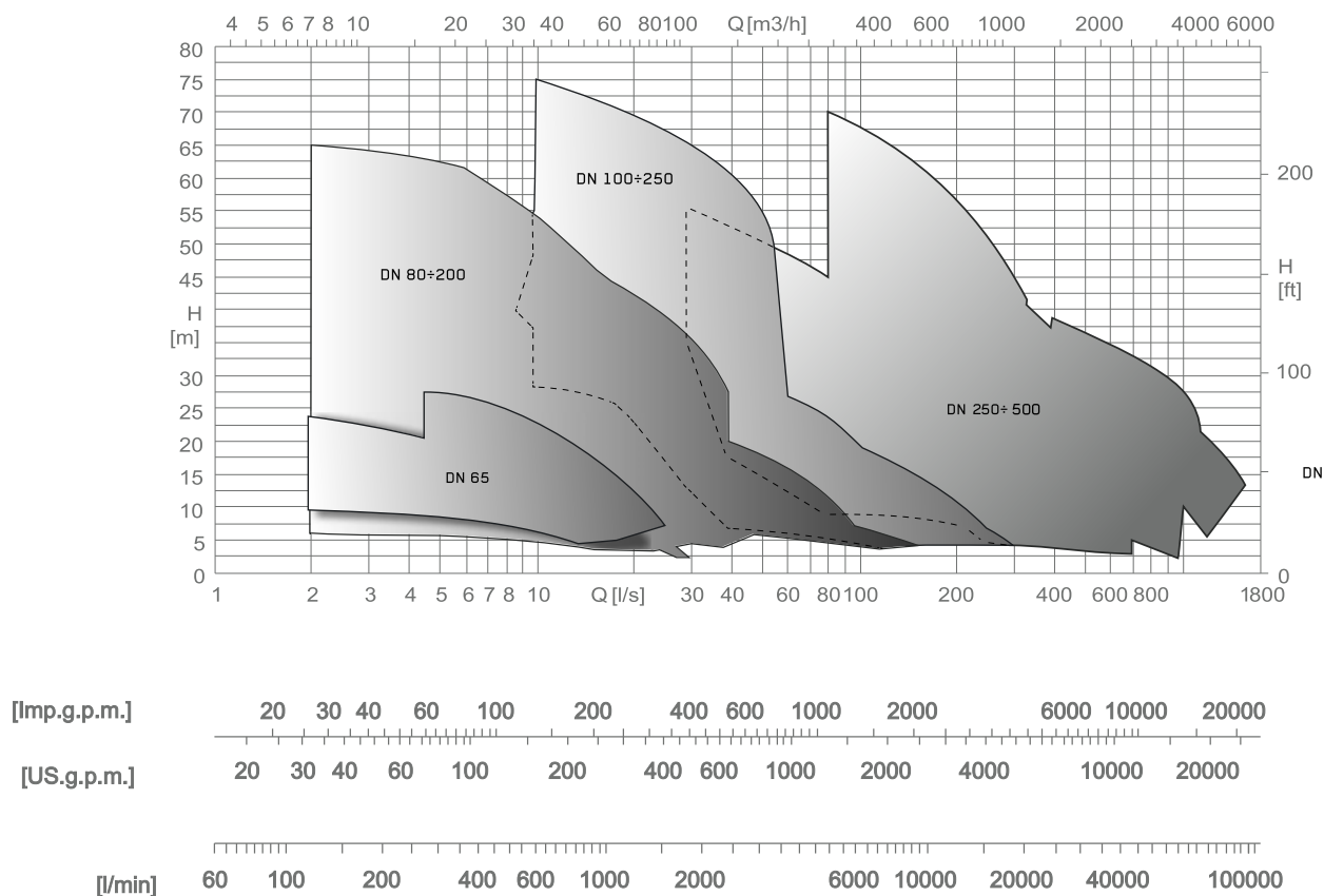
Campo de prestaciones Leistungsbereich Campo di prestazioni
