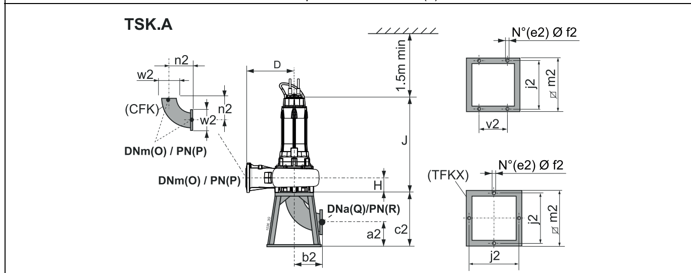
Version para cámara seca - vertical (/R) Für Trockeninstallation - senkrecht (/R) Esecuzione per camera asciutta - verticale (/R)
