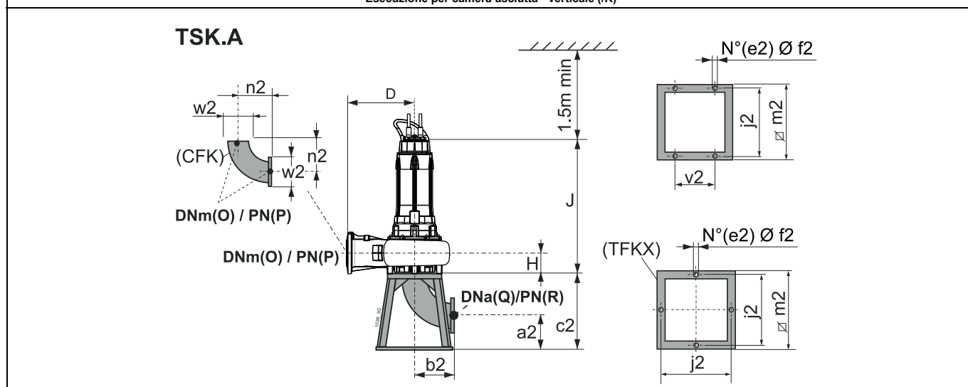
Versión para cámara seca - vertical (I/R) Für Trockeninstallation - senkrecht (I/R) Esecuzione per camera asciutta - verticale (I/R)
