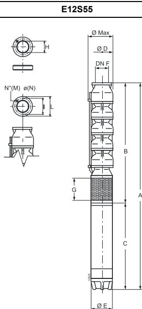
Overall dimensions and weights / Dimensions d'encombrement et poids Dimensioni di ingombro e pesi
