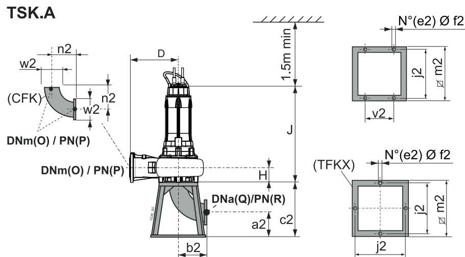
Versión para cámara seca - vertical (I/R) Für Trockeninstallation - senkrecht (I/R) Esecuzione per camera asciutta - verticale (I/R)
