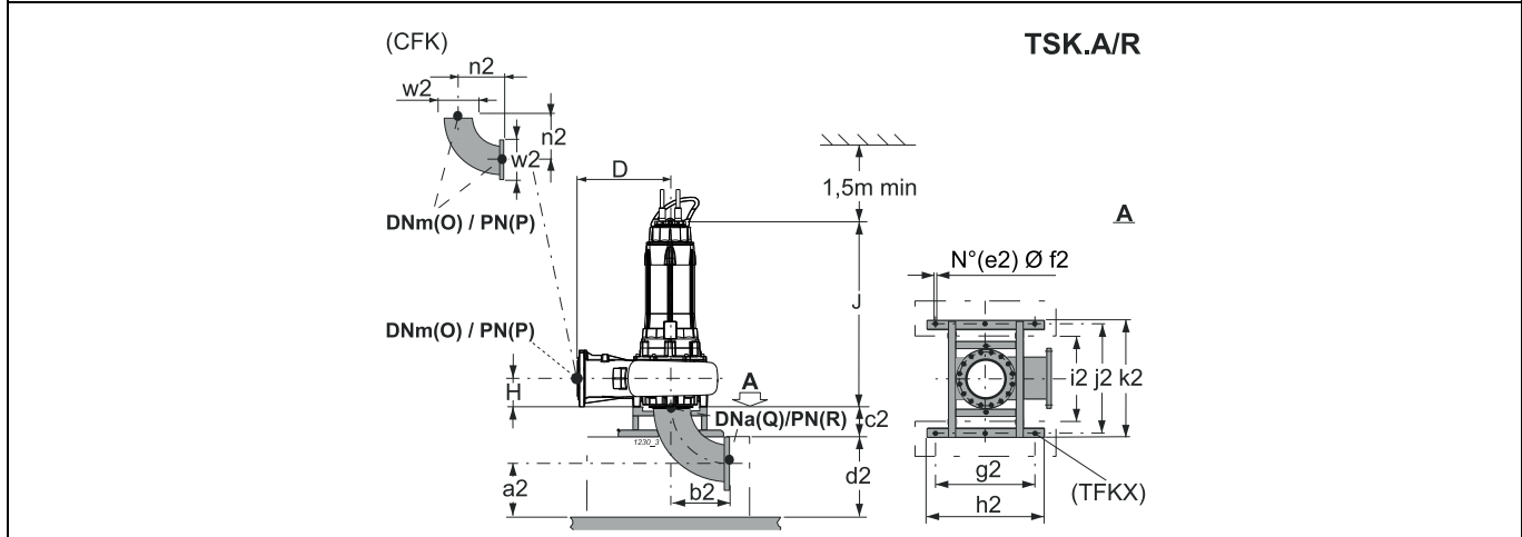
For fixed installation in a dry chamber - vertical (R) / Pour installation fixe en fosse sèche - verticale (R) / Esecuzione per camera asciutta - verticale (R)
